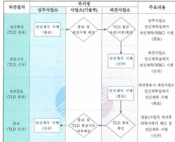
붙임1-(1). 원자력발전소 방사선관리구역 출입절차 흐름도(상주→국내파견)
